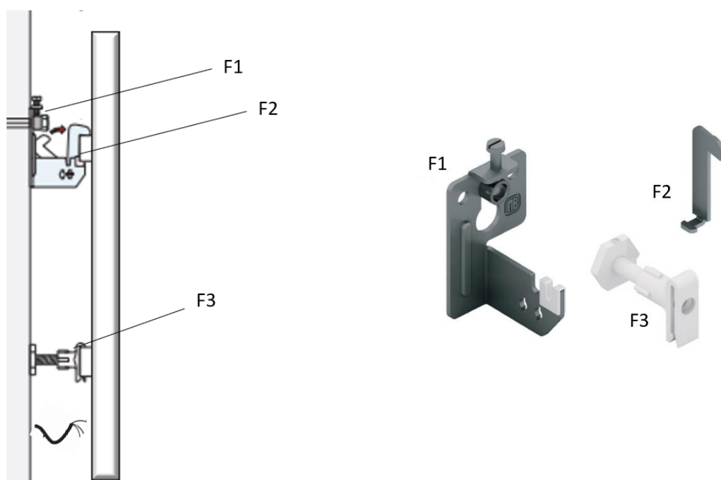
Vista laterale del termoarredo
