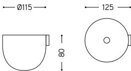
R4-1 Rosone ad una uscita Ceiling rose with one output
