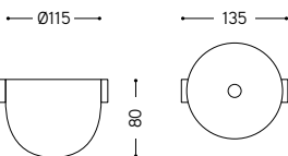
R4-180° Rosone con due uscite a 180° Ceiling rose with two 180° outputs
