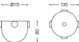
R4-4 Rosone decentramento con quattro uscite Shifted light point with four outputs
